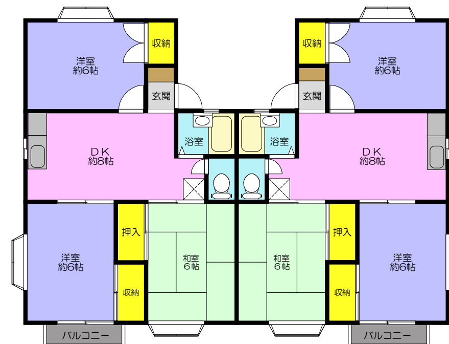
A棟 2階平面図
