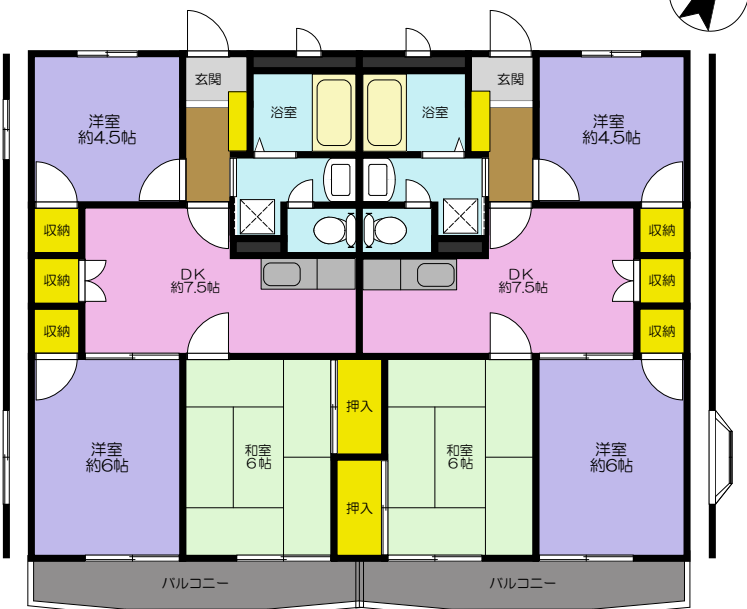
2階平面図
