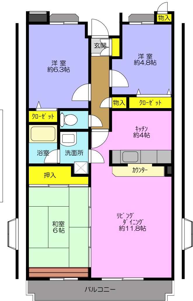
2階平面図
