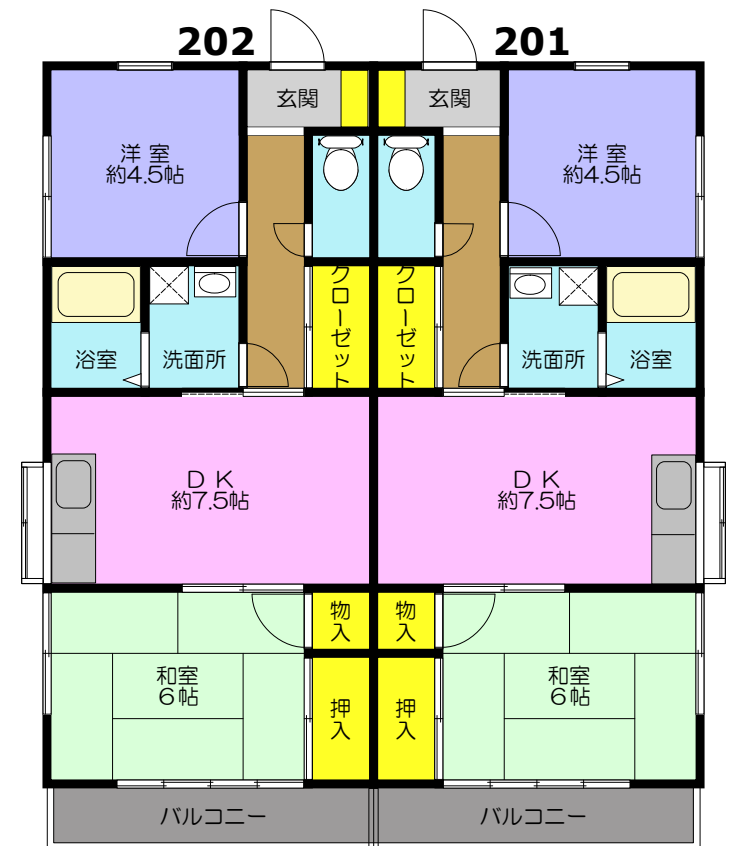
2階平面図
