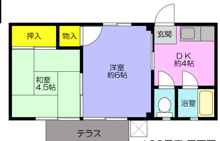
102号室 平面図
