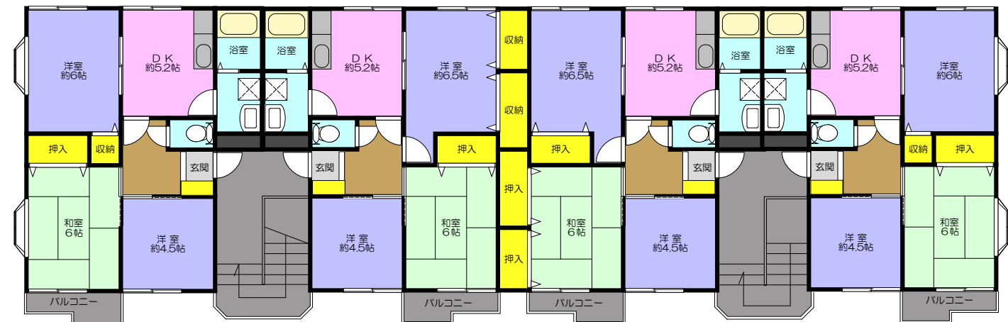
2階平面図
